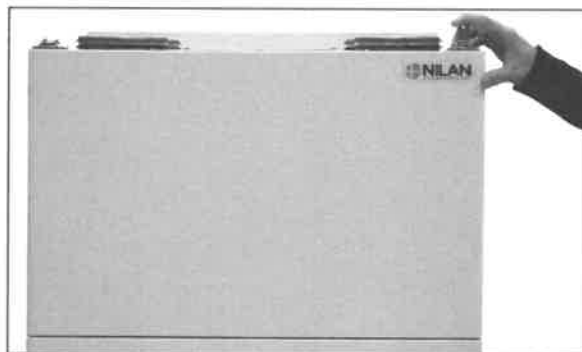
2. Kuffertbeslagene løsnes i den øverste låge og lågen løftes ud
